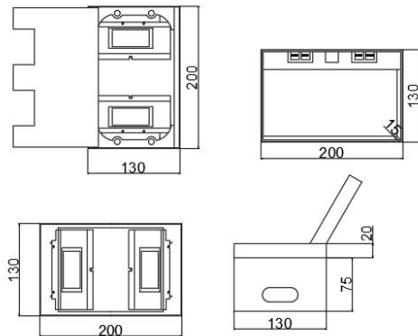
HTD-200B-CKP
