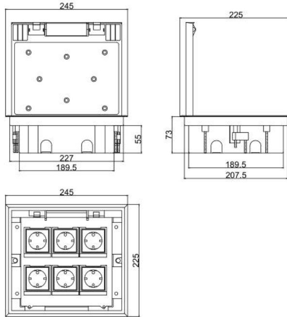
Units:mm
