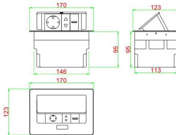
Units:mm
